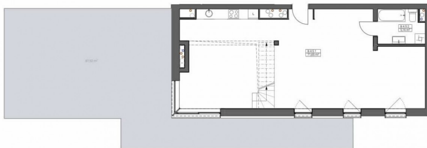
Piętro +4
