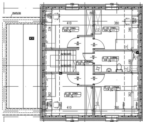
PODDASZE
