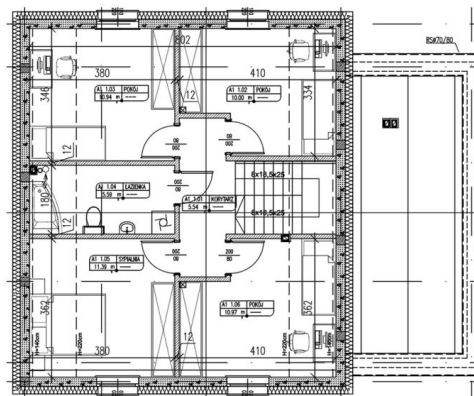
PODDASZE
