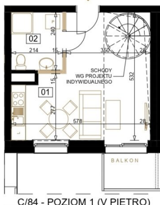
C/84 - POZIOM 1 (V PIĘTRO)
