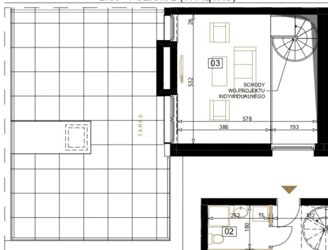
B/33 - POZIOM 2 (VI PIĘTRO)
