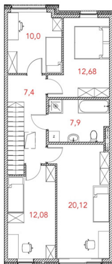
RZUT PIĘTRA
