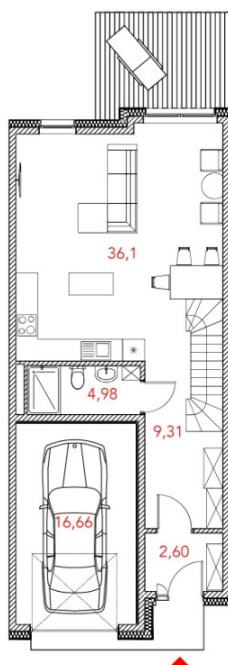
RZUT PARTERU
