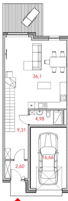
RZUT PARTERU
