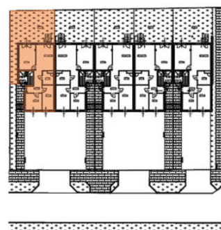
RZUT GARAŻY
