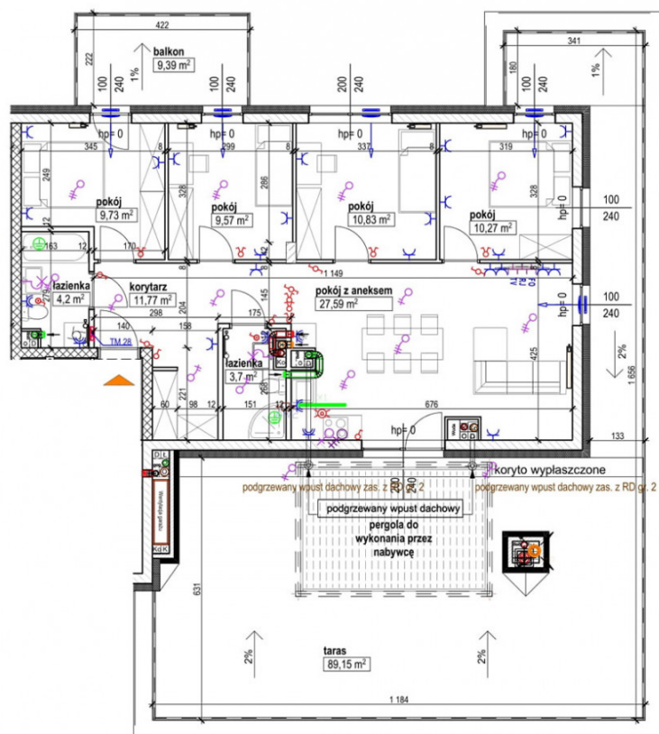
RZUT 2 PIĘTRA
