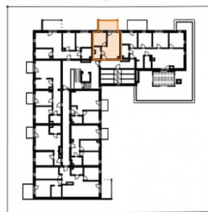
RZUT 2 PIĘTRA
