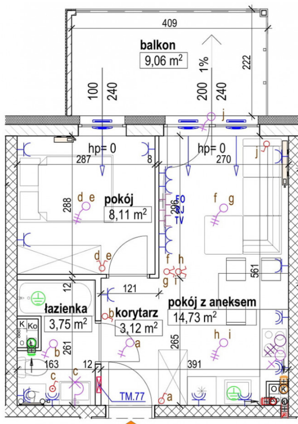
RZUT 2 PIĘTRA
