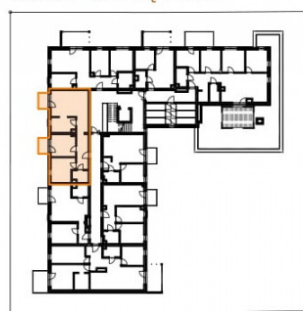
RZUT 2 PIĘTRA
