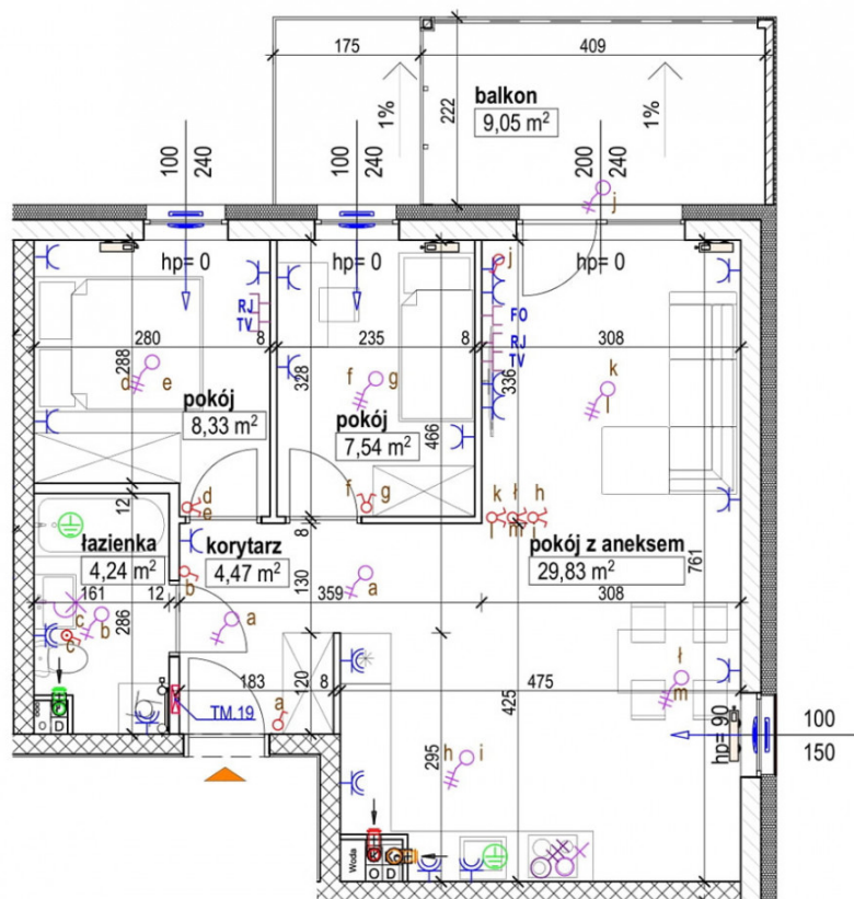
RZUT 1 PIĘTRA
