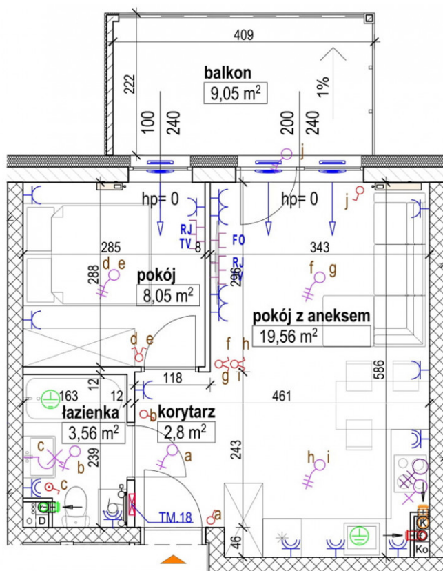
RZUT 1 PIĘTRA
