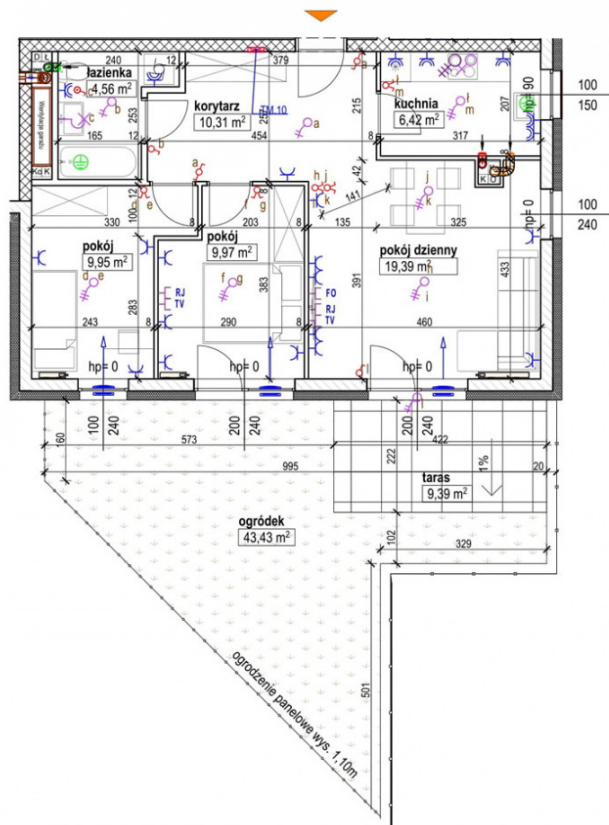
RZUT PARTERU
