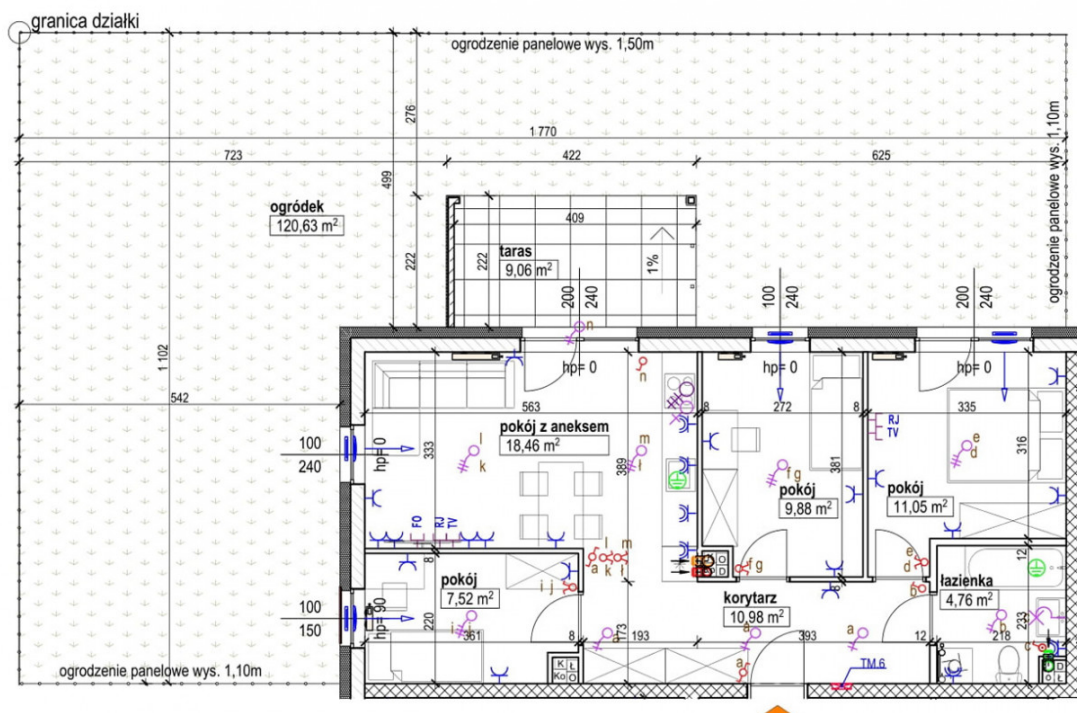
RZUT PARTERU
